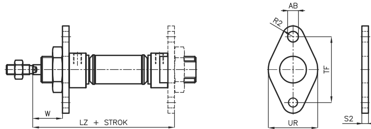
FB : Flanş Bağlantı / Flange Mounting
