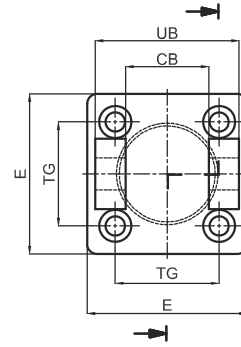
IÇB: Çatal Bağlantı Piston rod clevis mounting
