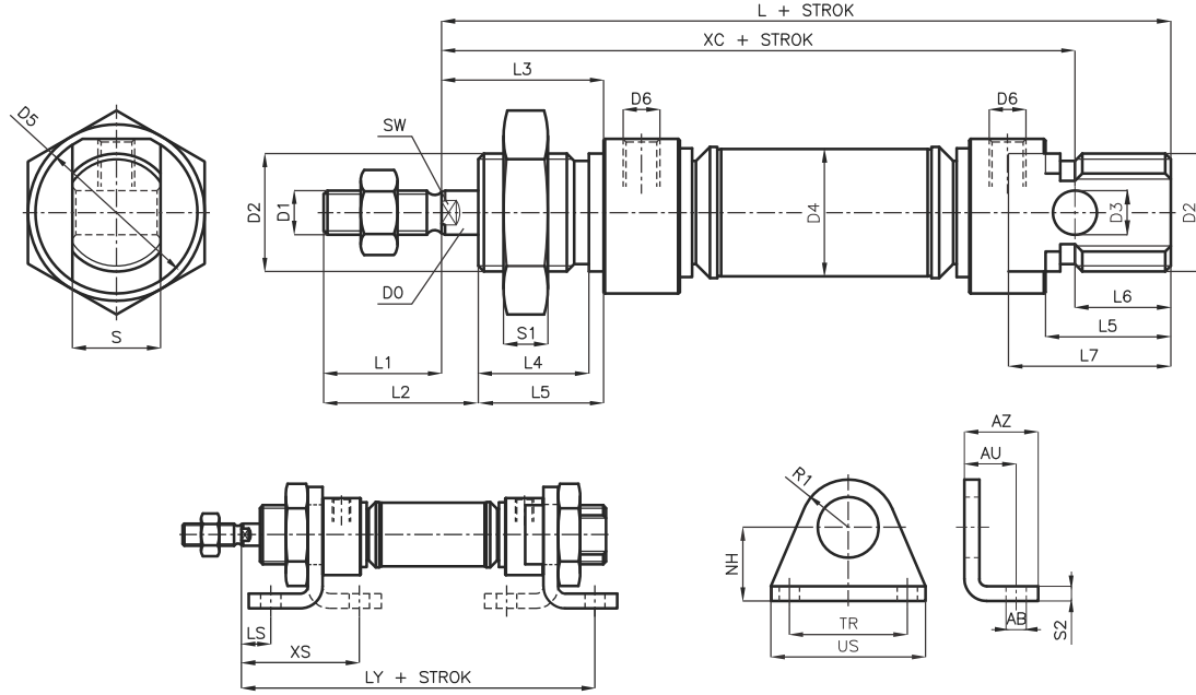
AB : Ayak Bağlantı / Foot Mounting
