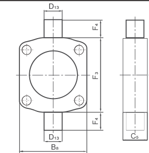
OEB: Orta eklem bağlantı Trunnion mounting
