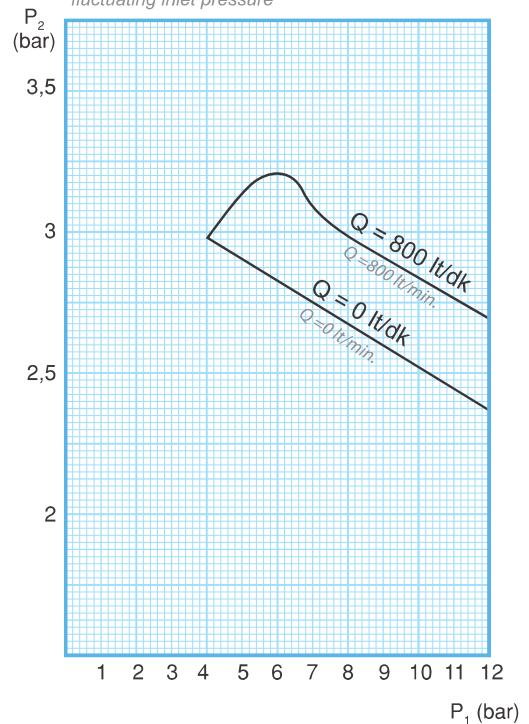
Giriş basıncına bağımlılık eğrisi
