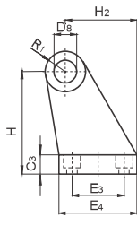
YB: Yer bağlantı Clevis foot
