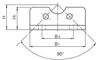
AB: Ayak bağlantı Foot mounting
