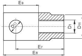
ÇB: Çatal bağlantı Piston rod clevis mounting
