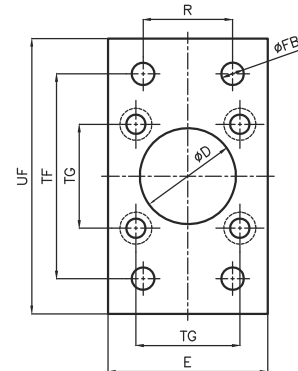
IEB: Eklem bağlantı Swivel flange mounting
