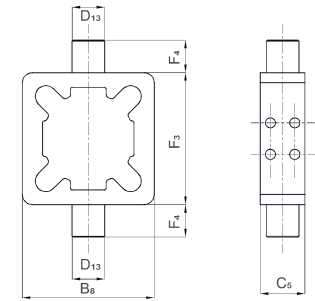
ÖEB: Orta eklem bağlantı Trunnion mounting
