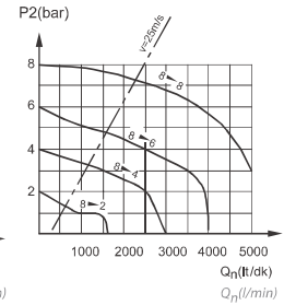
Akış Özellikleri (M(FR)Y 1/2) Flow characteristics (M(FR)Y 1/2)
