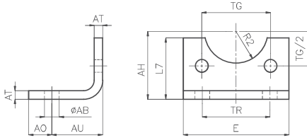
IAB: Ayak bağlantı Foot mounting
