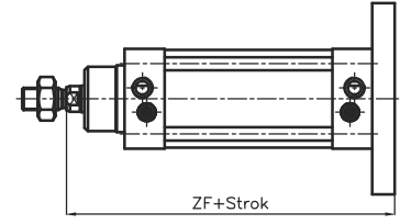
Arka flanş bağlantı Rear flange mounting
