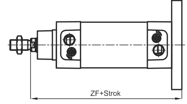
Arka flanş bağlantı Rear flange mounting
