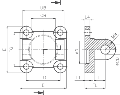
IEB: Eklem bağlantı Swivel flange mounting
