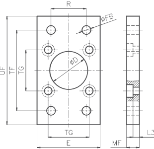
IFB: Flanş bağlantı Flange mounting
